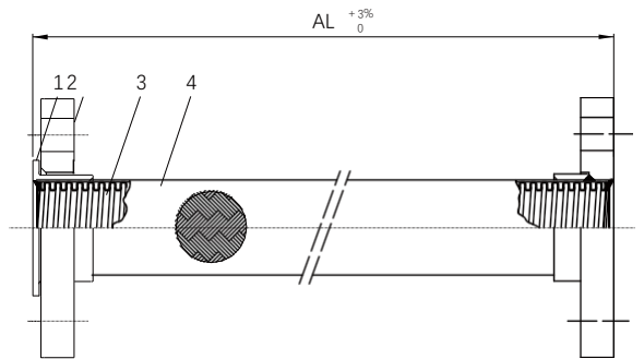
一端固定型
